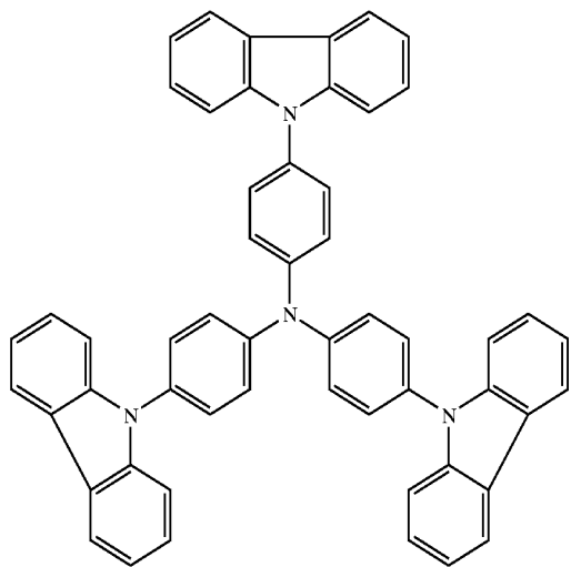
TCTA ( T_g = 101^\circ \text{C.} )
