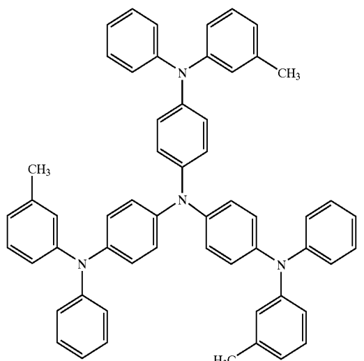
m-MTDATA ( T_g = 75^\circ \text{C.} )
