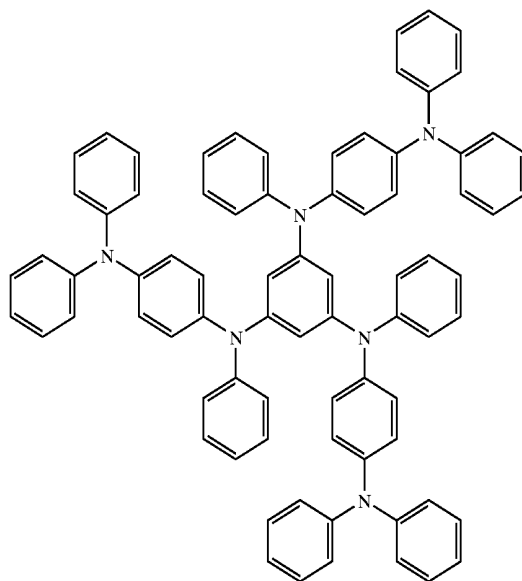
p-DPA-TDAB ( T_g = 108^\circ \text{C.} )
